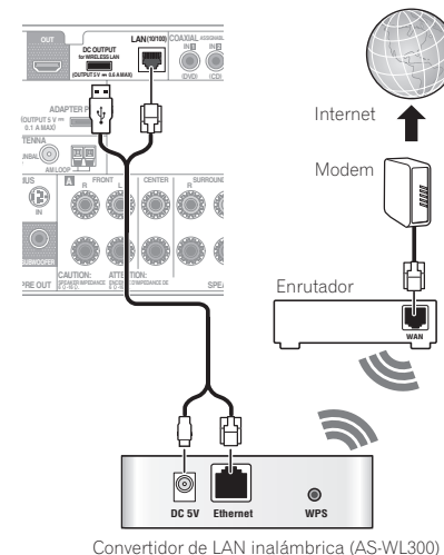
Convertidor de LAN inalámbrica (AS-WL300)
